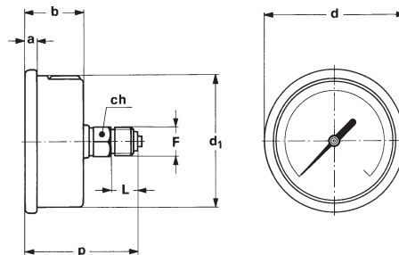
TIPO D per montaggio locale diretto su tubazione; con raccordo posteriore.
