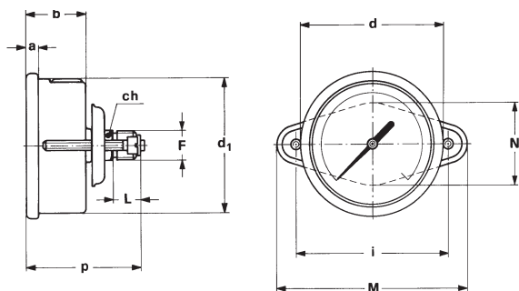
TIPO B per montaggio a pannello; con staffa e raccordo posteriore.
